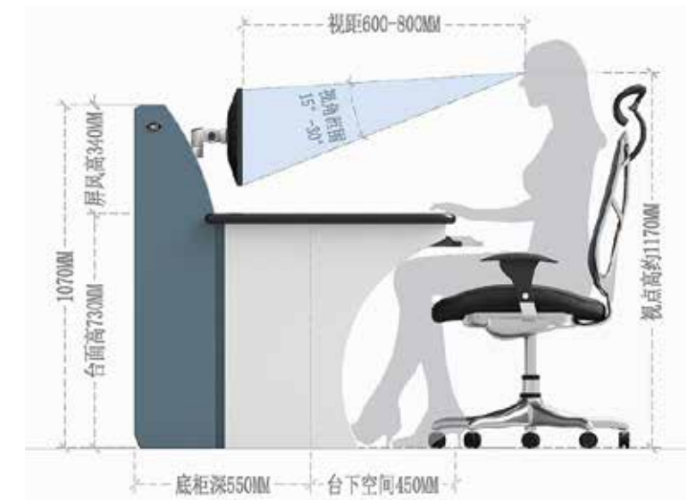
Ideal work station (for reference) 操作台给使用者理想工作空间 (只供参考)
